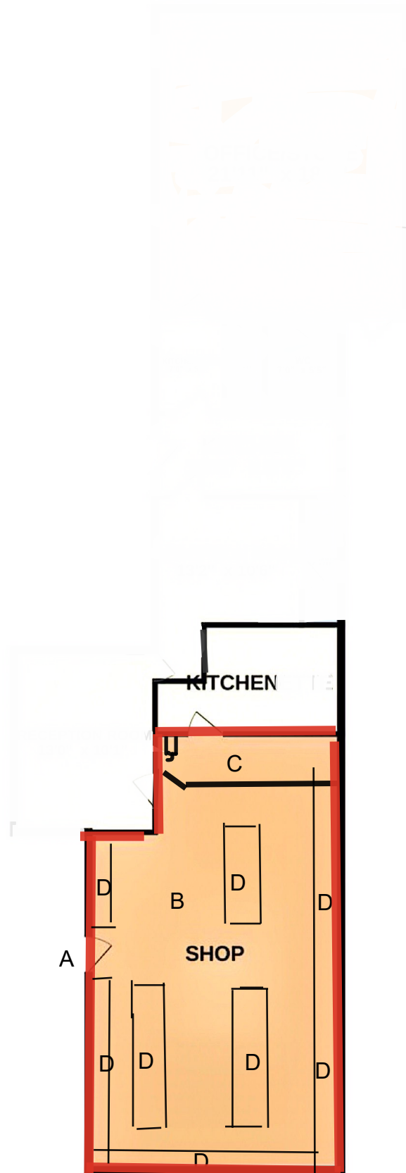
PREMISES PLAN 1:100
